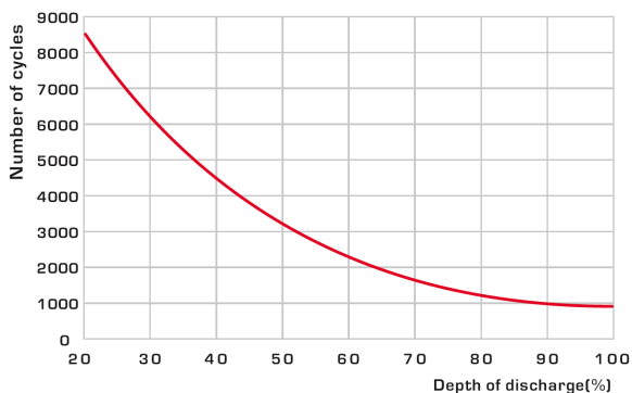
Bild 13. Lebensdauer in Abhängigkeit von der Entladetiefe
